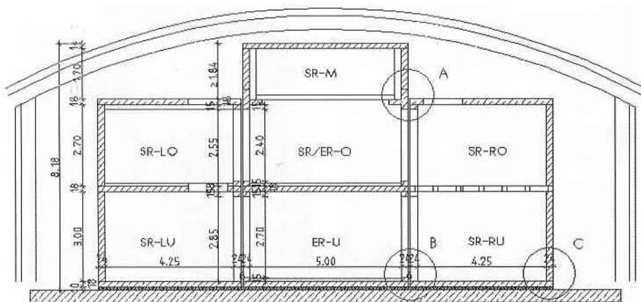
Querschnitt durch das neue Treppenprüfzentrum
